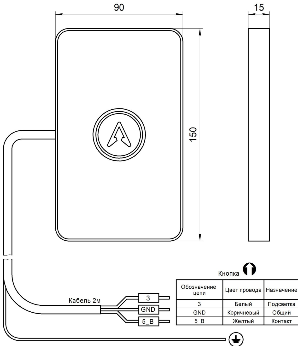
Рис.1 Внешний вид и габаритные размеры Вызывного поста ОНИКС НШЕК.468381.123
